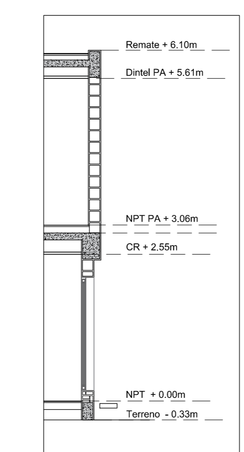
DETALLE CONSTRUCTIVO
